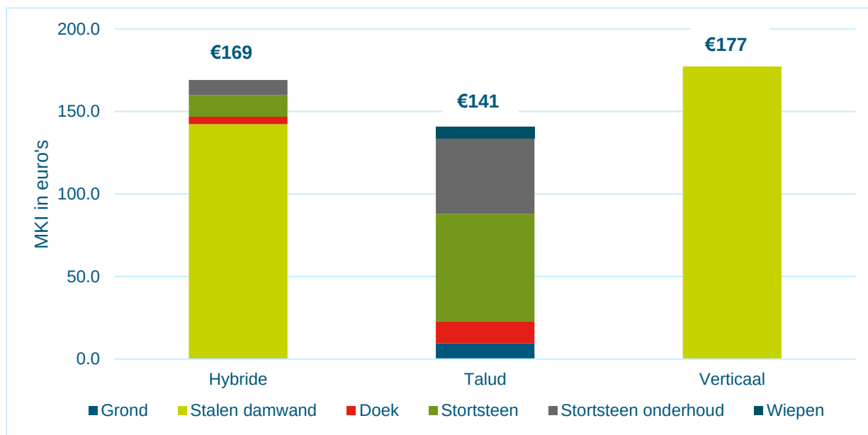
Figuur 9: Zwaartepuntanalyse per principe-oplossing voor profiel A bij gemiddelde invoerwaarden. De belangrijkste onderdelen van de MKI-waarden worden zichtbaar.
